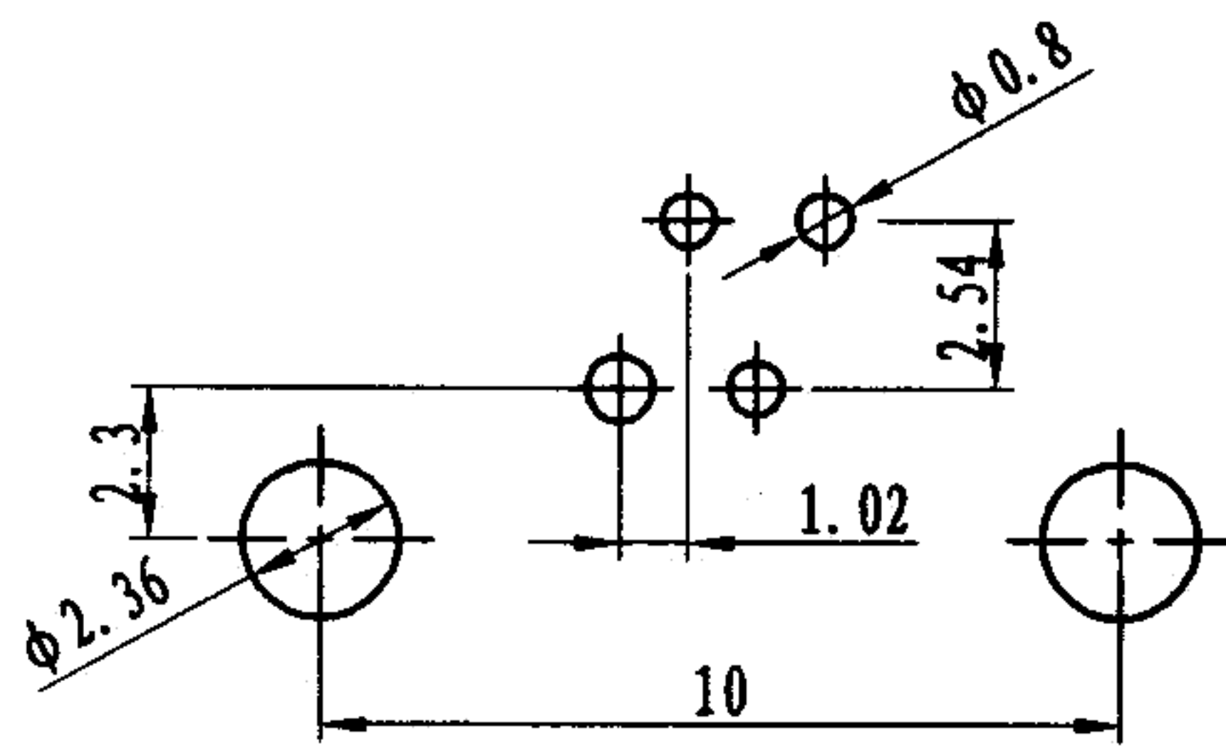
PC 板孔位
