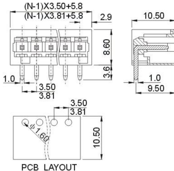
8EDGRC-3.5 8EDGRC-3.81
